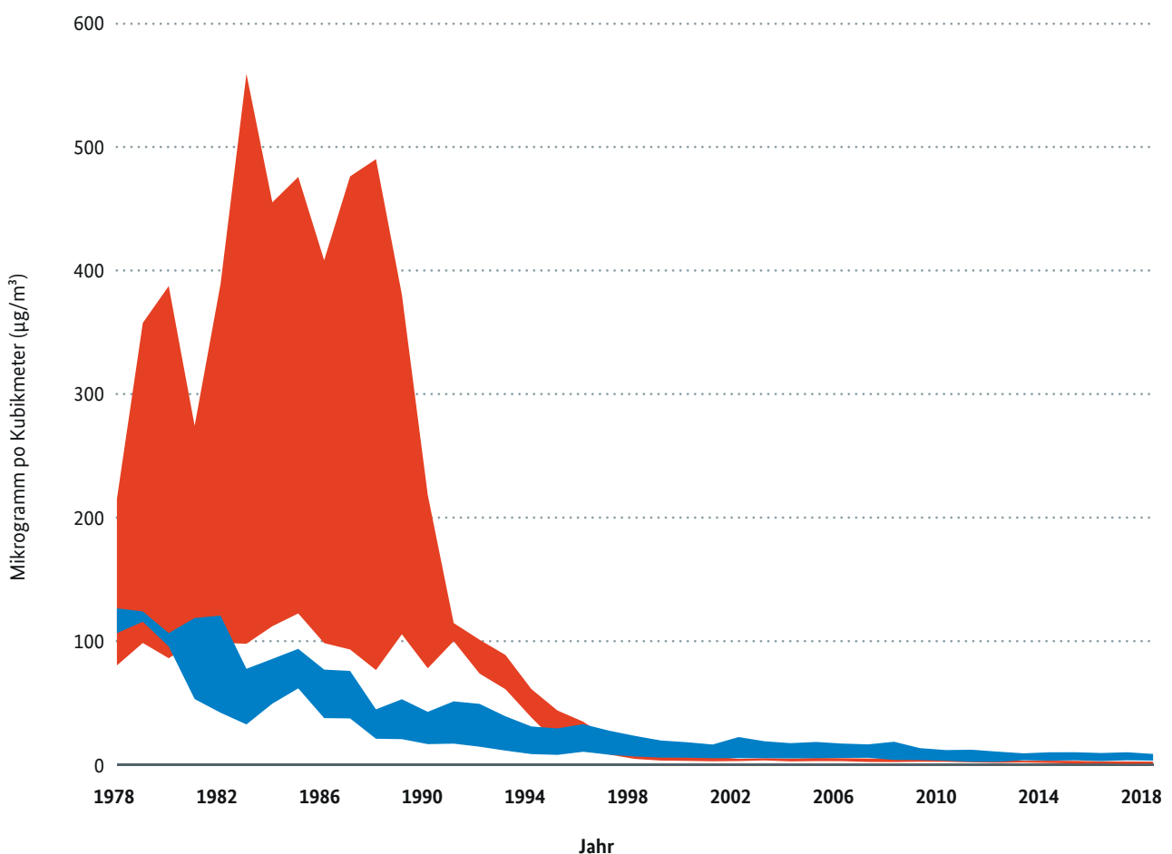
Abbildung 73: SO 2 -Jahresmittelwerte
